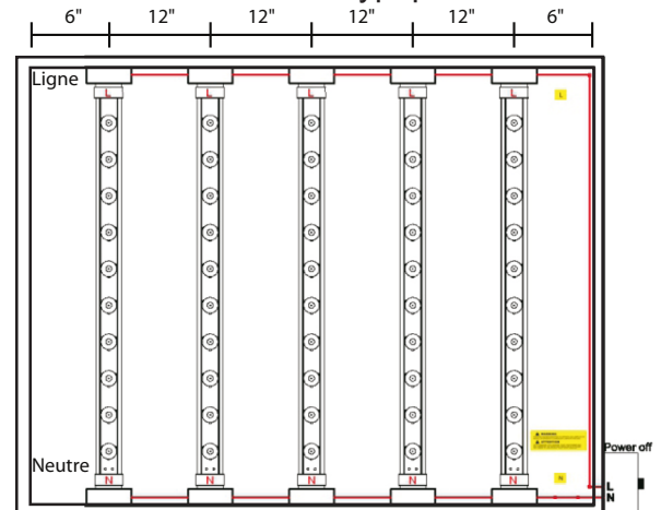
Installation typique
